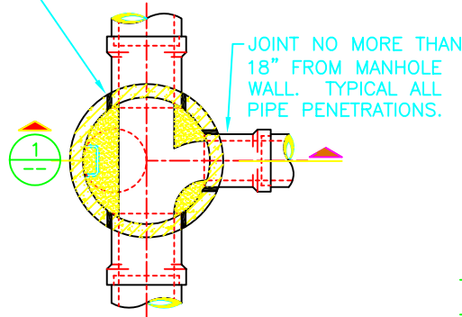
CAST IN PLACE BASE JOINT (D) -- SCALE: NTS
