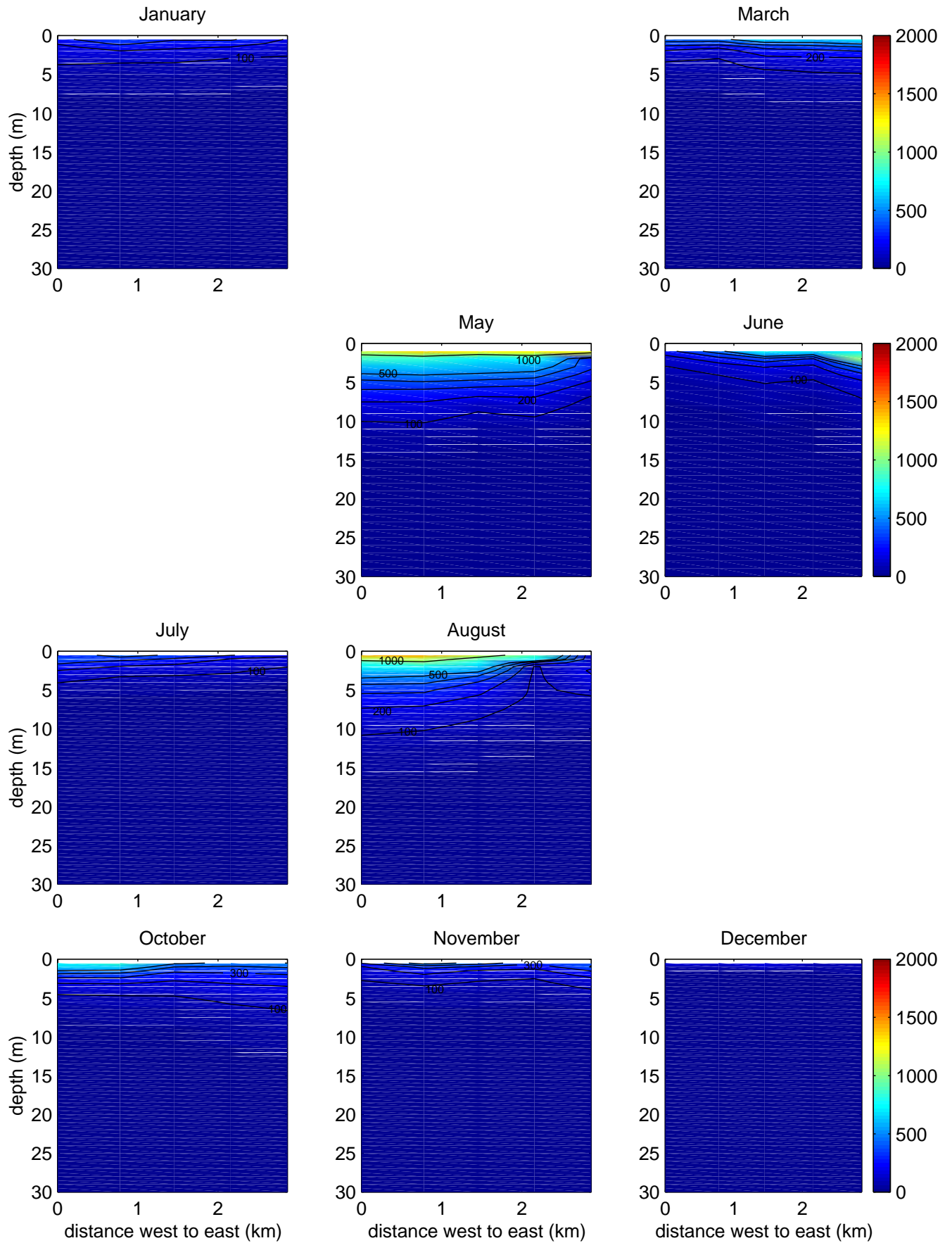
Figure 4-45. Possession PAR ( \mu\text{mol}/\text{sm}^2 ) 1999
